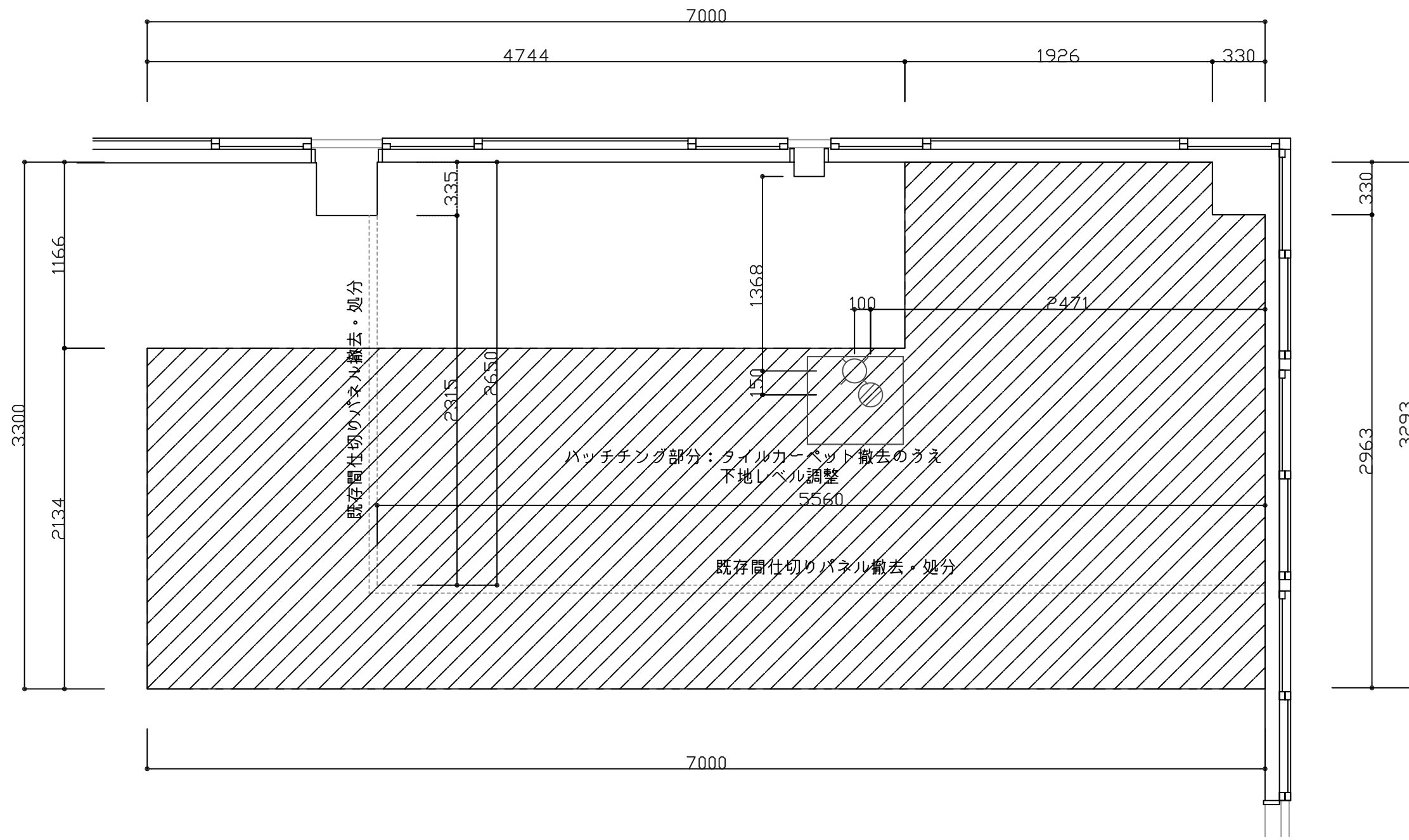
既存改修 平面図 S = 1 / 30
